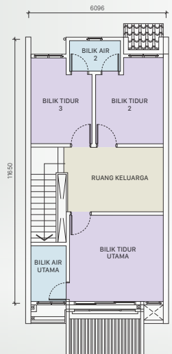
PLAN LANTAI ARAS SATU
