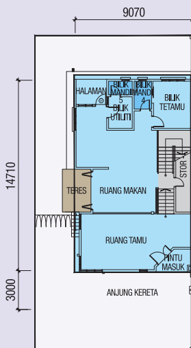
PELAN LANTAI TINGKAT BAWAH
