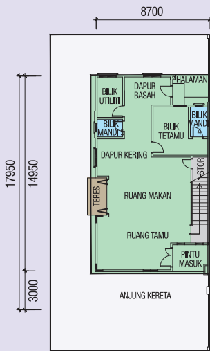
PELAN LANTAI TINGKAT BAWAH
