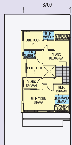
PELAN LANTAI TINGKAT ATAS
