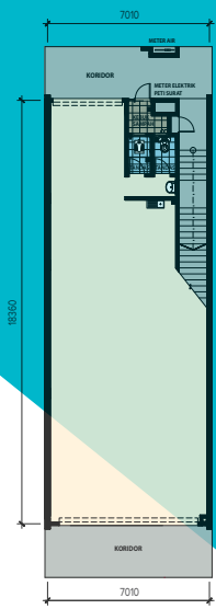
PELAN LANTAI ARAS BAWAH
